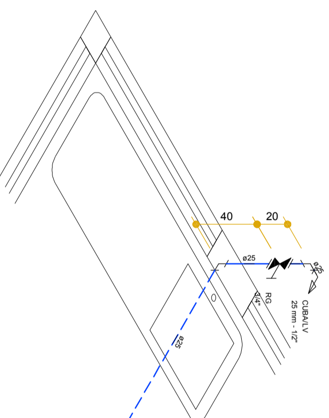
DETALHE H4 ESCALA 1/25
