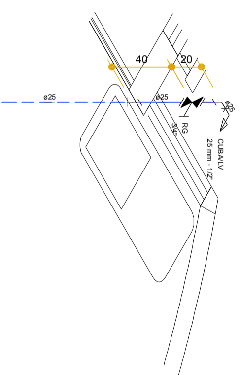
DETALHE H2 ESCALA 1/25
